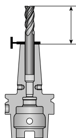
Werkzeug auf Anschlag einführen. Futter abkühlen lassen bis Werkzeug gespannt wird.
