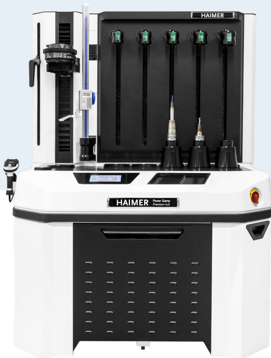
Abbildung zeigt PC407422-C11-EU mit Längenvoreinstellung und Scanner (optional) Picture shows PC407422-C11-EU with length presetting and scanner (optional)
